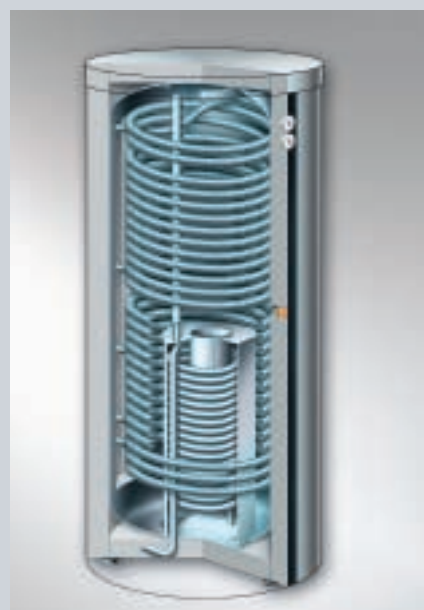
Fig. 36 : Réservoir tampon d'eau primaire multiénergie Vitocell 360-M à système de charge et de production d'eau chaude intégrée
