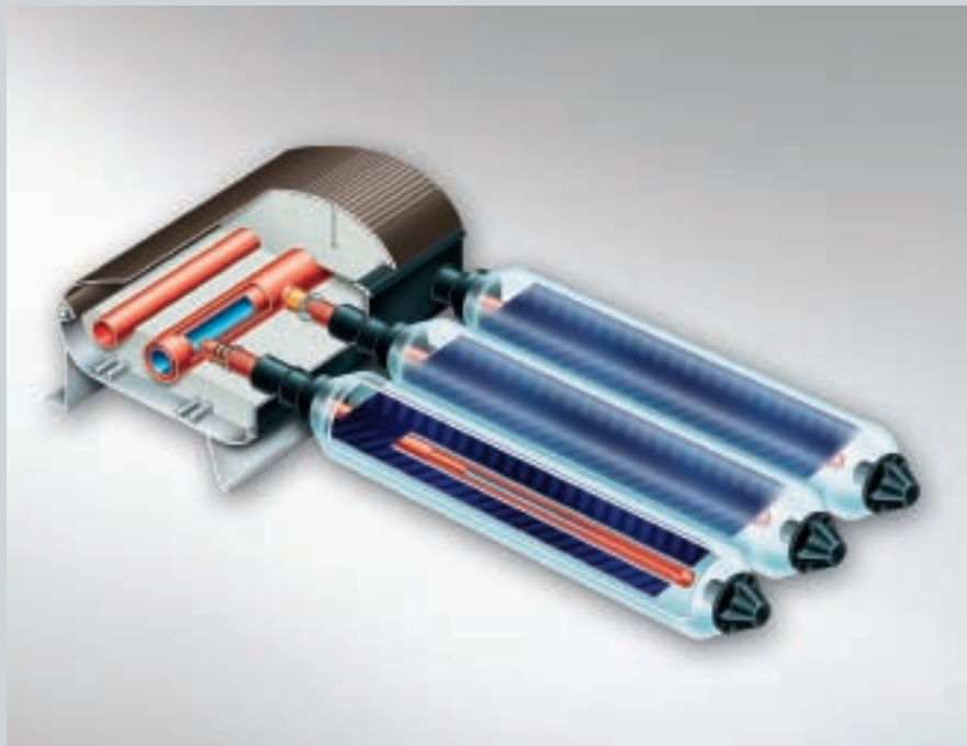
Fig. 22 : Capteur solaire à tubes sous vide Vitosol 200-T
