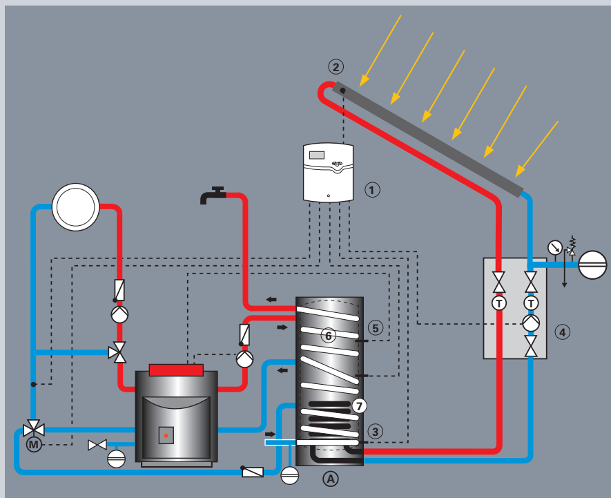
Fig. 43 : Production d'eau chaude sanitaire bivalent et appoint du chauffage avec des capteurs solaires et une chaudière
