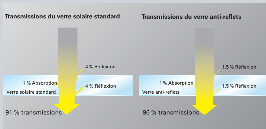
Fig. 19 : Transmissions du verre solaire standard et du verre anti-reflets
