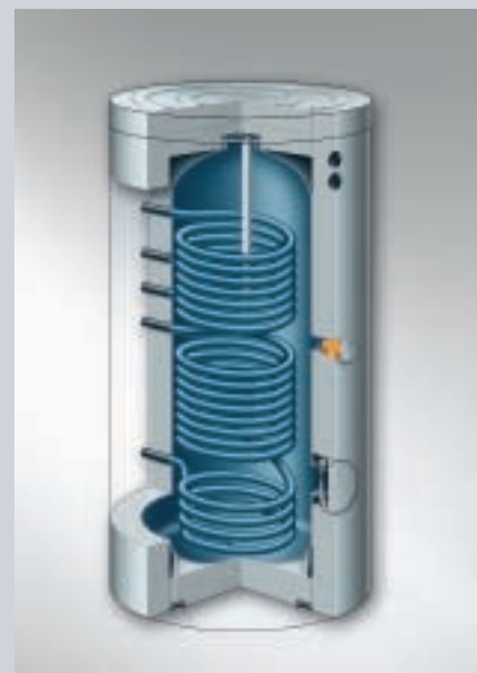
Fig. 27 : Ballon d'eau chaude bivalent Vitocell 100-B en acier et à émailage Céraprotect (400 et 500 litres de capacité)
