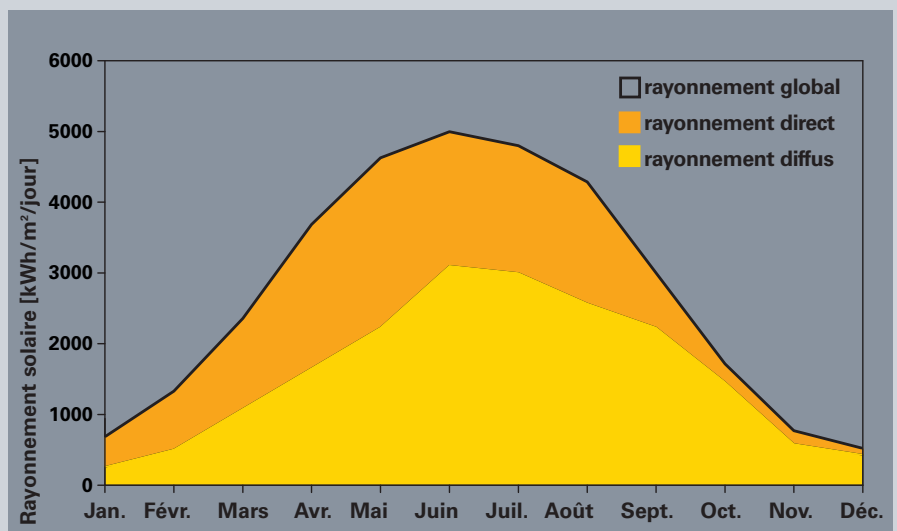
Fig. 3 : Puissance rayonnée quotidiennement par le soleil sur une année
