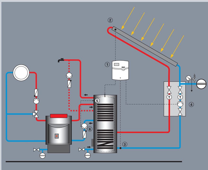
Fig. 41 : Production d'eau chaude sanitaire bivalent avec des capteurs solaires et un préparateur d'eau chaude sanitaire deux énergies
