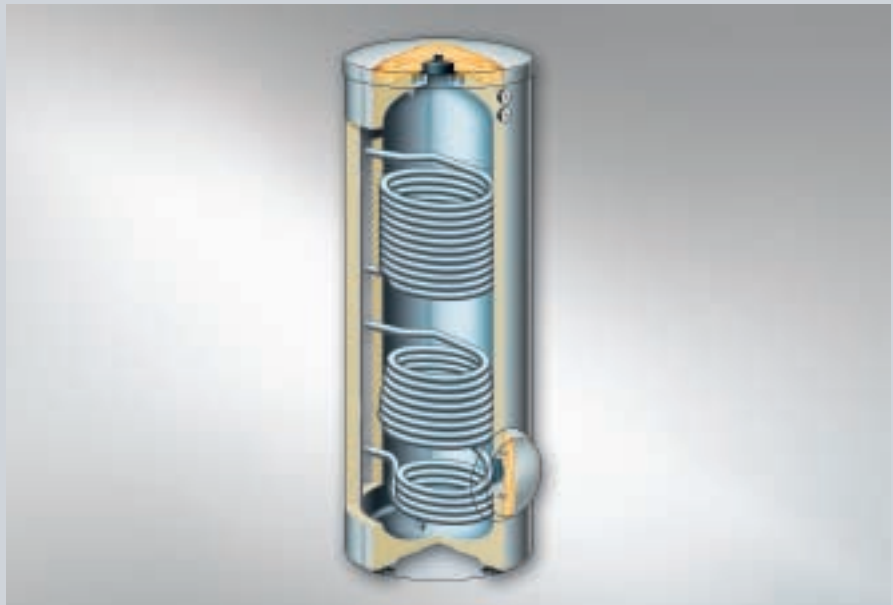
Fig. 30 : Ballon d'eau chaude bivalent Vitocell 300-B en acier inoxydable austénitique
