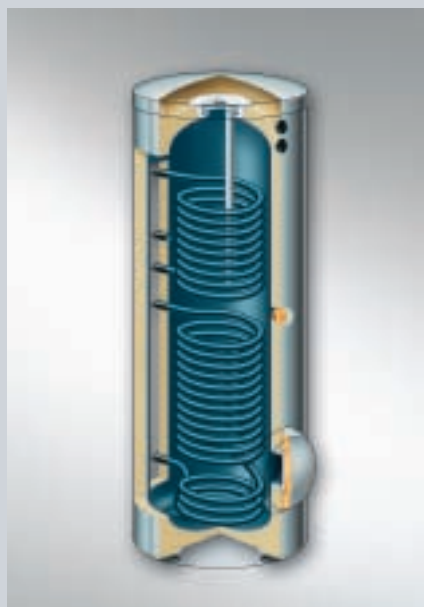
Fig. 26 : Ballon d'eau chaude bivalent Vitocell 100-B en acier et à émailage Céraprotect (300 litres de capacité)
