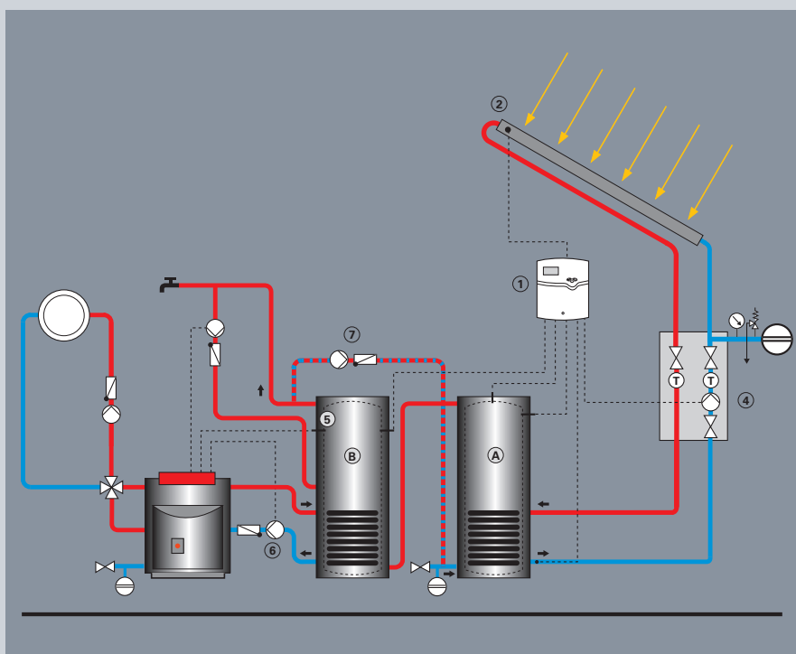
Fig. 42 : Production d'eau chaude sanitaire bivalent avec des capteurs solaires et deux préparateurs d'eau chaude sanitaire
