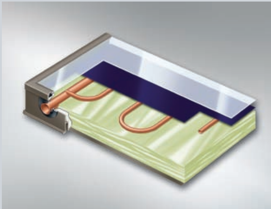
Fig. 18 : Capteur solaire plan Vitosol 200-F
