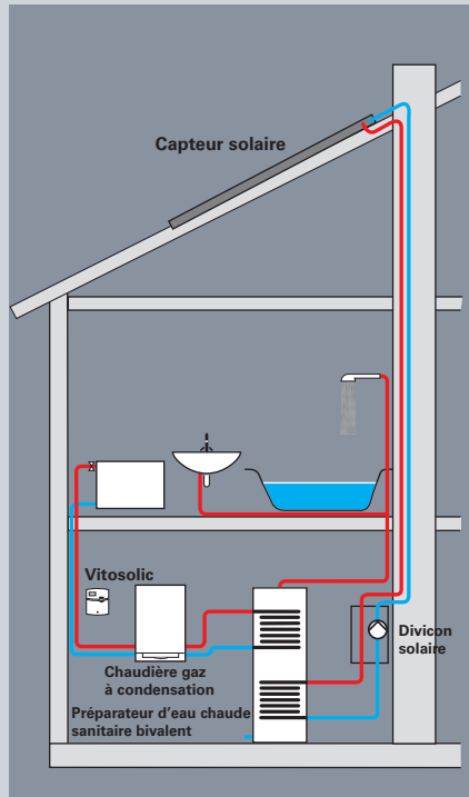
Fig. 37 : Installation solaire Viessmann associée à une chaudière gaz à condensation et à un préparateur d'eau chaude sanitaire bivalent
