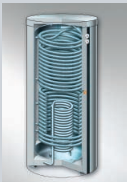
Fig. 35 : Réservoir tampon d'eau primaire multiénergie Vitocell 340-M à production d'eau chaude intégrée
