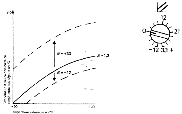
Fig. 20 Réglage du parallèle de la courbe de fonctionnement du circuit de chauffage
