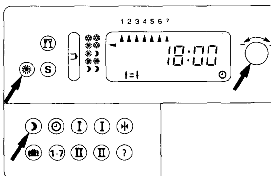
Fig. 15 Réglage des consignes de température ambiante sur la commande à distance-F
