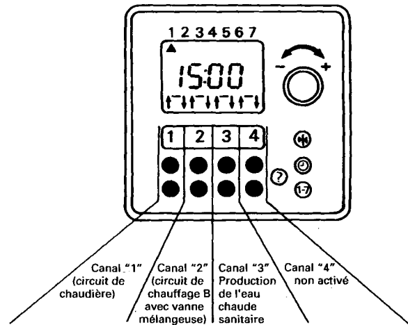
Fig. 5 Horloge numérique Affectation des canaux
