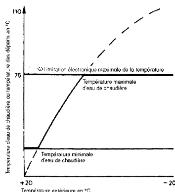
Fig. 22 Exemple de courbes de fonctionnement réglées
