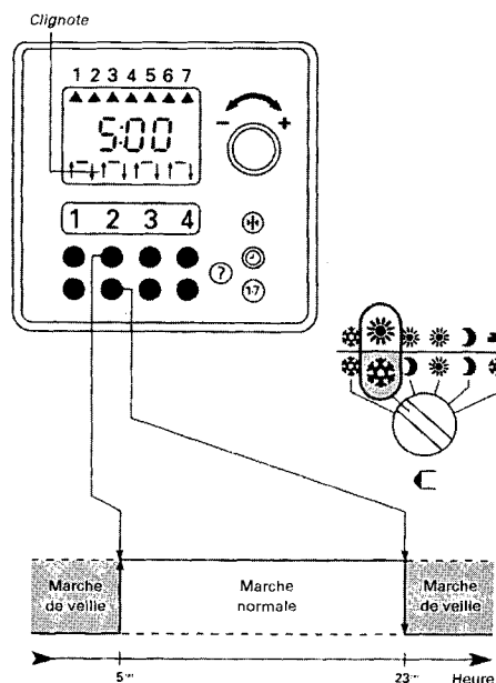
Dans l'exemple représenté, - la séquence "rouge" correspond à la marche normale - la séquence "bleue" correspond à la marche de veille avec mise hors gel
