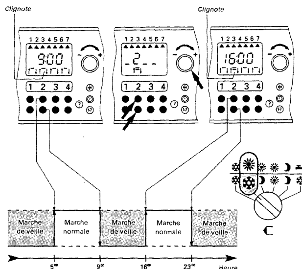
Dans l'exemple représenté, - la séquence "rouge" correspond à la marche normale - la séquence "bleue" correspond à la marche de veille avec mise hors gel
