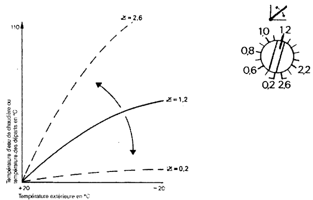
Fig. 19 Sélection de la courbe de fonctionnement du circuit de chauffage
