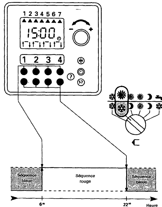
Fig. 6 Programmation de base de l'horloge (canal "2", par exemple)
