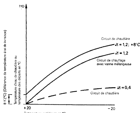
Fig. 21 Courbe de température d'eau de chaudière
