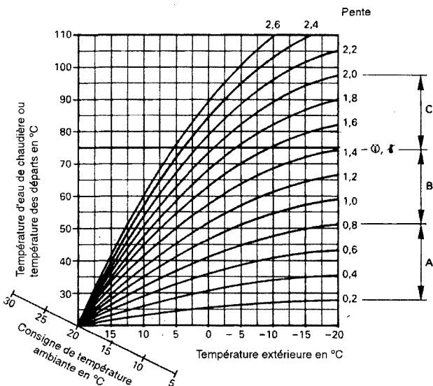
Fig. 18 Courbes de fonctionnement sélectionnables (Valeurs indicatives pour les températures d'eau de chaudière ou des départs moyennes)
